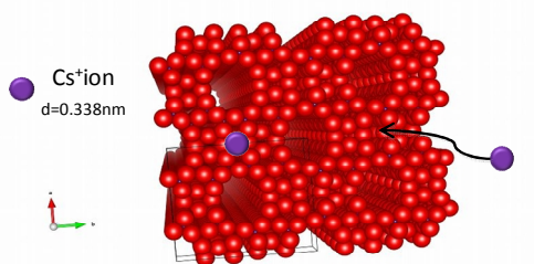
図 4. モルデン沸石へのセシウムイオンの吸着モデル図 11)
