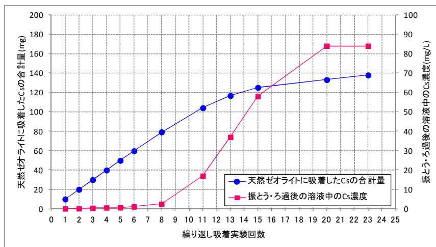
図8. 繰り返し吸着実験結果グラフ
