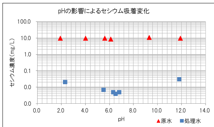
図 6. ゼオライトに対するセシウムの吸着実験結果グラフ
