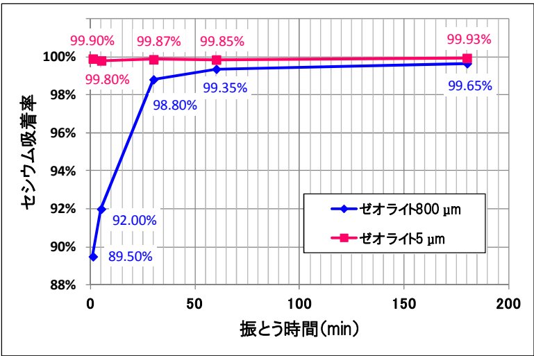
図 7. ゼオライト粒度毎のセシウム吸着実験結果グラフ
