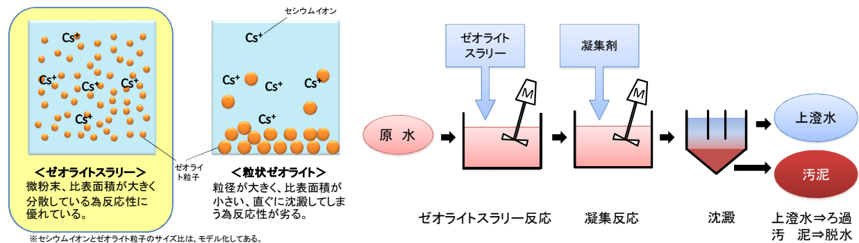
(左) 図 9. ゼオライトスラリーと粒状ゼオライトの効果比較概念図
