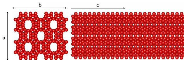
図 2. モルデン沸石 c 軸方向伸延モデル図 11)
