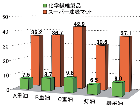
油の種類別による吸着量の比較（製品1g当たりの吸着量）
